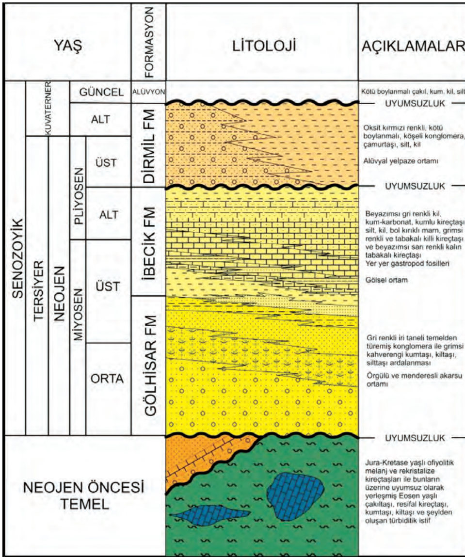
Şekil 3. Çalışma alanının stratigrafik kesiti (Elitez, 2010).
